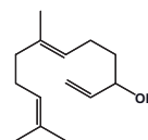
Nerolidol
